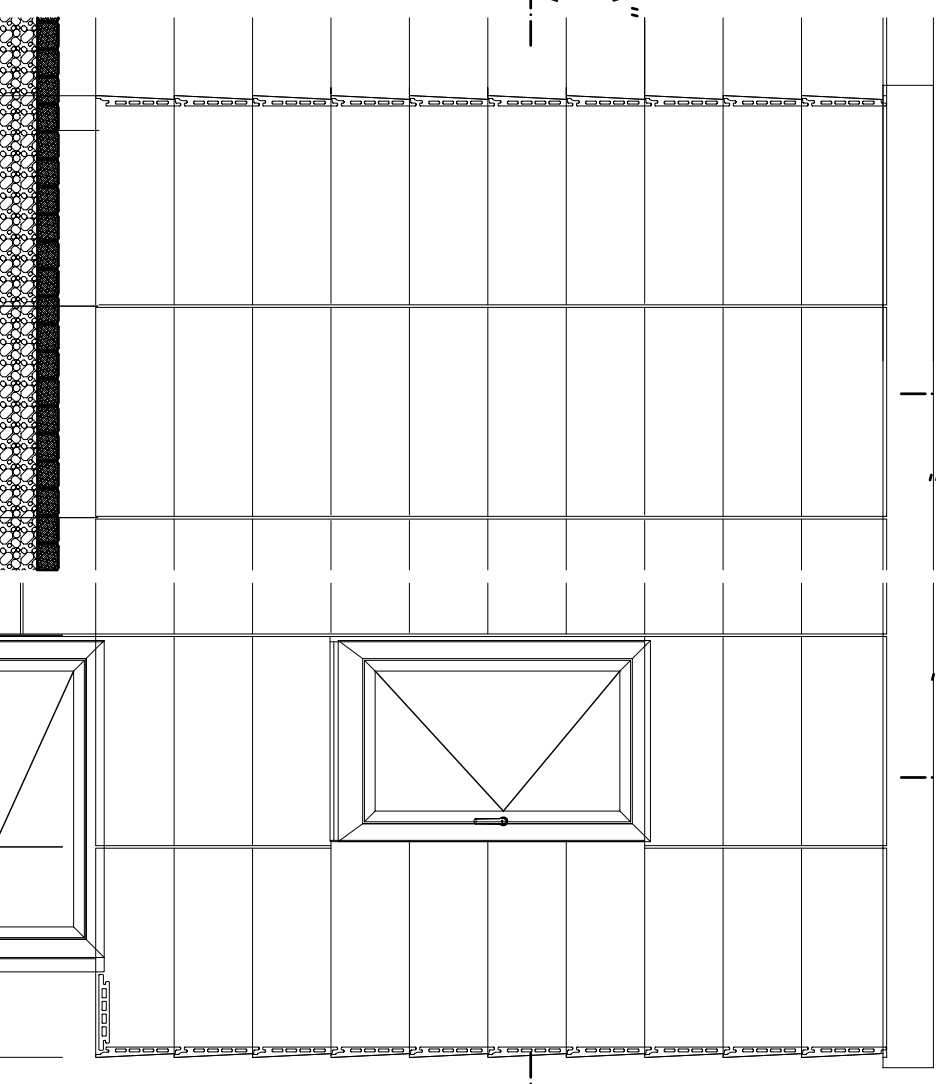
SCHNITT "A-A"
